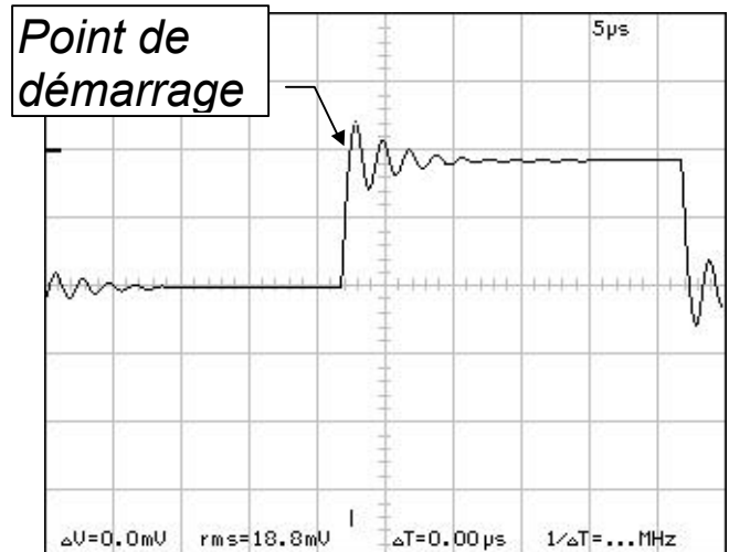
Fig 4. La fonction de pré-démarrage permet de visualiser le signal avant le démarrage.
