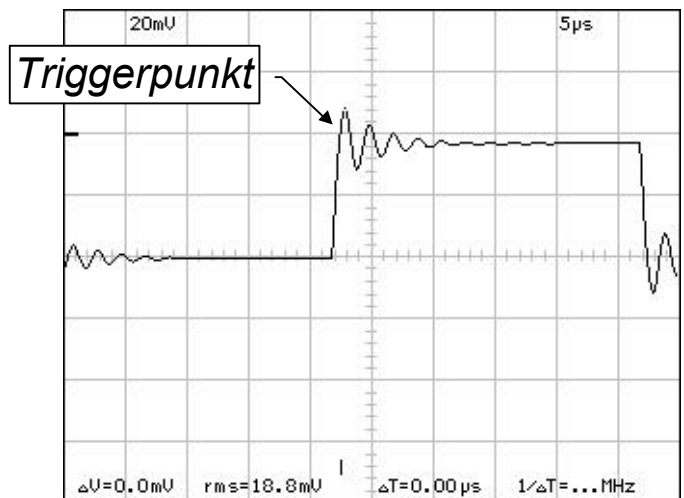
Fig 4. Pre-trigger-Funktion ermöglicht es, sich das Signal noch vor Triggering anzusehen.
