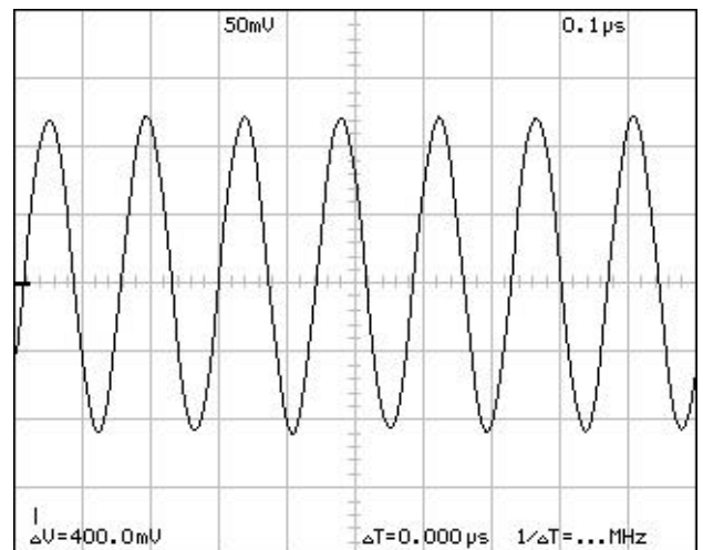
Abgerundete Interpolation
