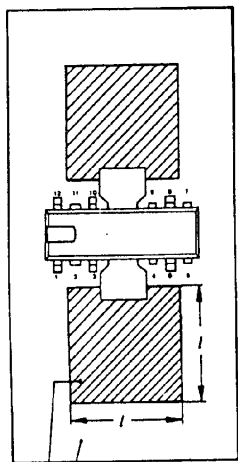
Fig. 4 Kupferfläche 35 \mu\text{m} dick Copper area 35 \mu\text{m} thickness
